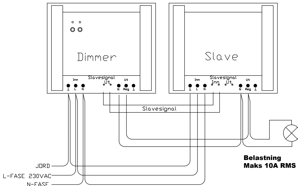
Koblingseksempel CENTROL CDIM(U)TS05 med slave
