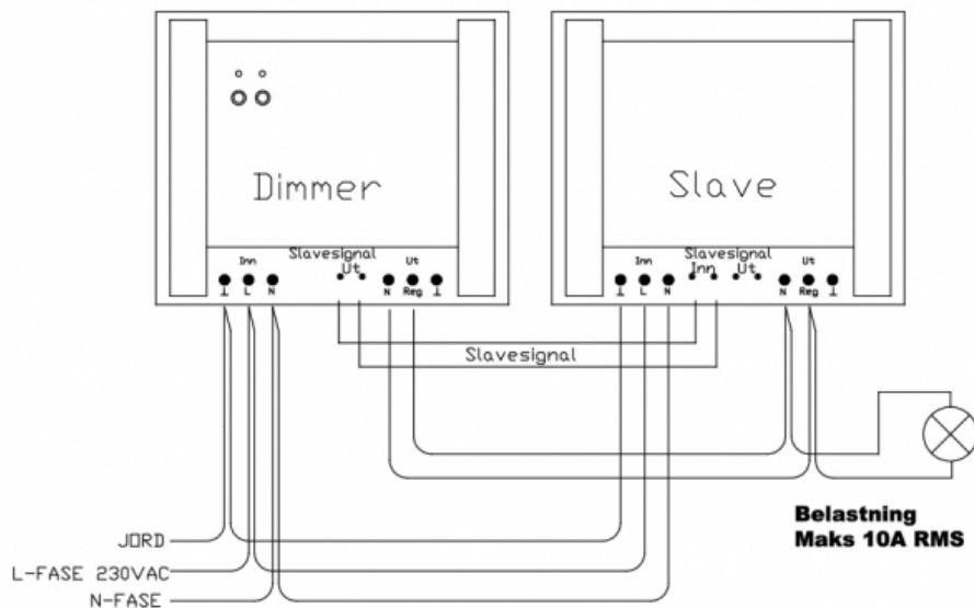
Koblingseksempel CENTROL CDIM(U)TS05 med slave
