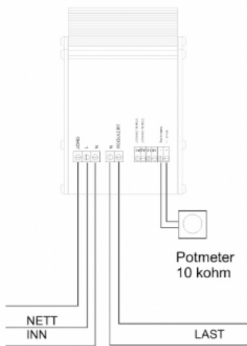
KOBLINGSEKSEMPEL MED POTMETERREGULERING
