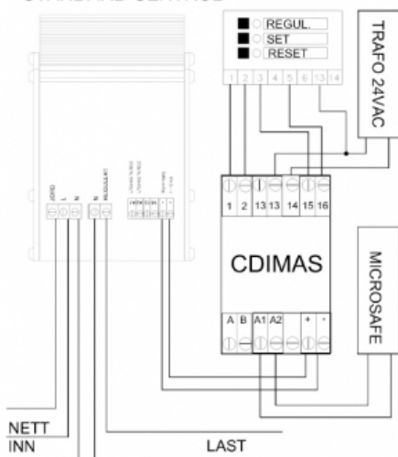
KOBLINGSEKSEMPEL SAMMEN MED STANDARD CENTROL
