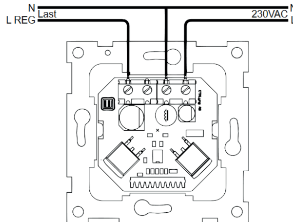
Kobling med felles N-leder:
